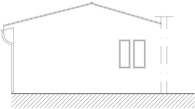
Prospetto Ovest C-C'
