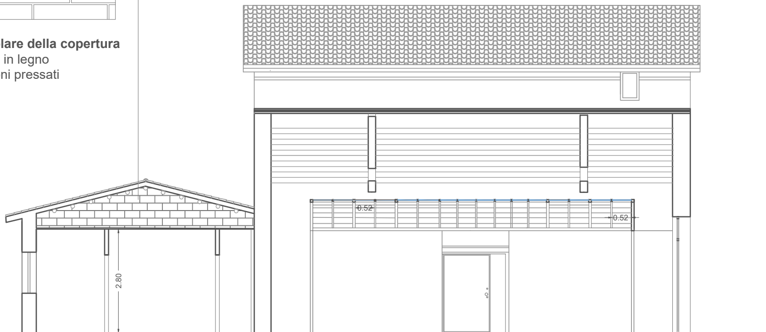
Sezione A-A'
