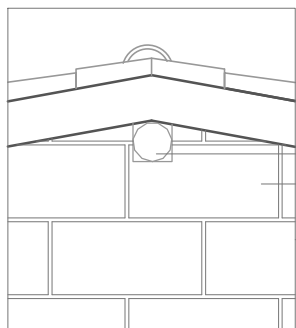
Particolare della copertura 1 Trave in legno 2 mattoni pressati
