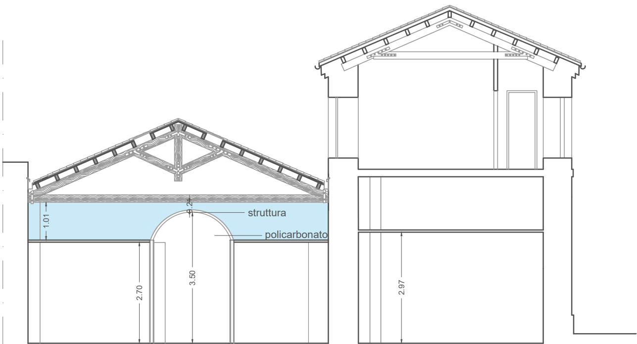
Sezione B-B'
