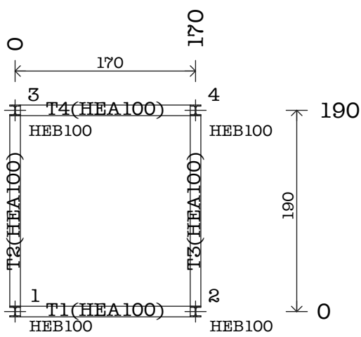
CARPEN. 3°SOLAIO QUOTA 9,20
