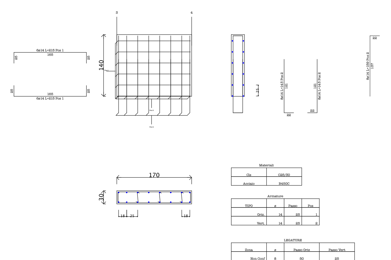
Parete non Dissipativa4 Piano 1 Fili Fissi 3-4
