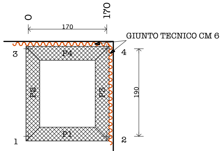
CARP. 1°SOLAIO QUOTA 1.40 mt.
