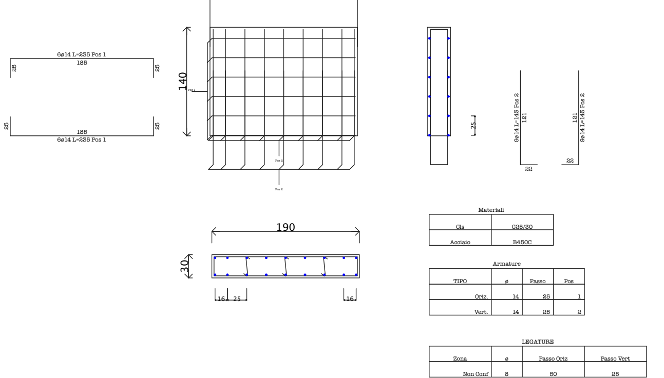
Parete non Dissipativa3 Piano 1 Fili Fissi 4-2
