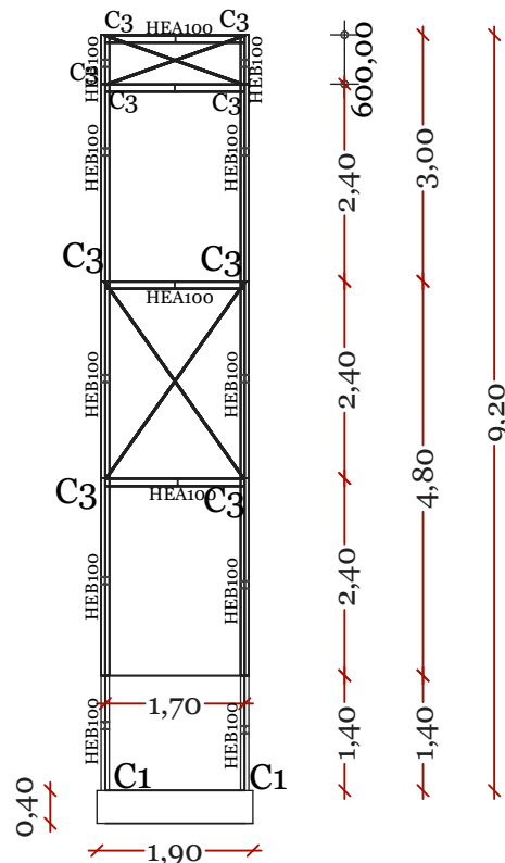
CONTROVENTI DI PARETE F20
