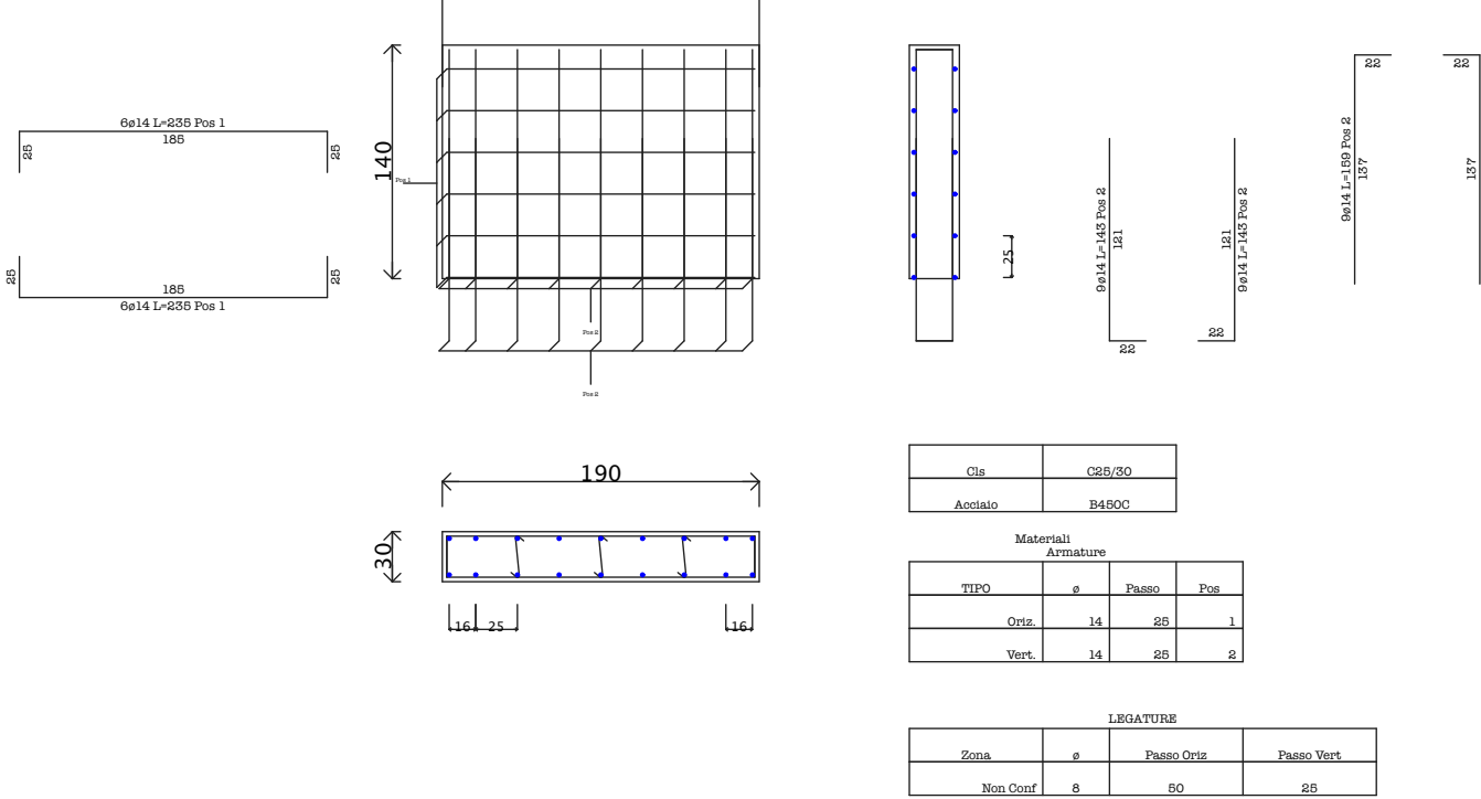
Parete non Dissipativa2 Piano 1 Fili Fissi 3-1
