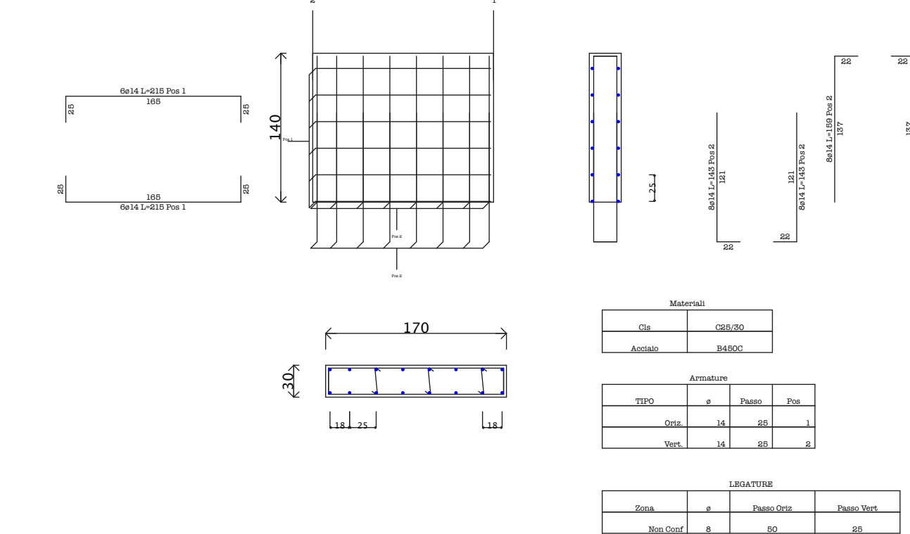
Parete non Dissipativa1 Piano 1 Fili Fissi 2-1
