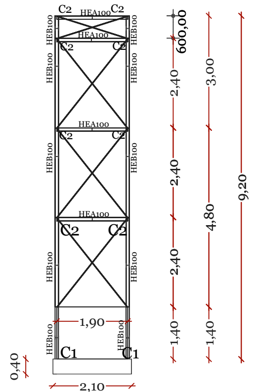
CONTROVENTI DI PARETE F20
