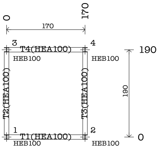
CARPEN. 2°SOLAIO QUOTA 6,20
